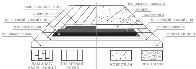
Рисунок 23. Схемы укладки твердых и мягких напольных покрытий.
