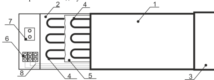
Рис. 1. Устройство обогревателя
