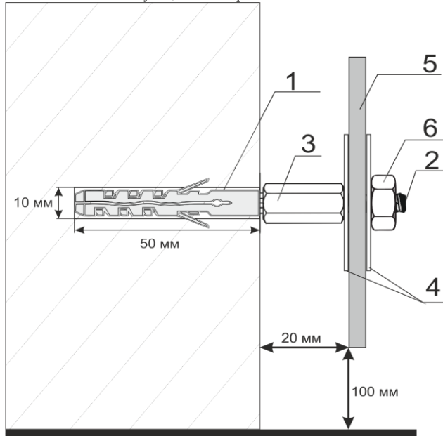
Рис. 2. Монтаж обогревателя
